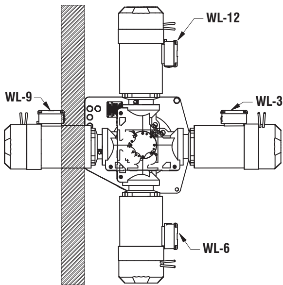
Wall Mount Left (WL)
